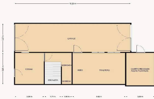
SÓTANO
